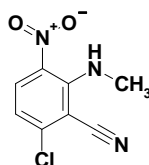
6-chloro-2-(methylamino)-3-nitrobenzenecarbonitrile
