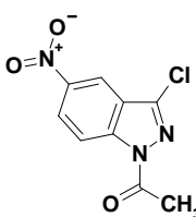
1-(3-chloro-5-nitro-1H-indazol-1-yl)-1-ethanone
