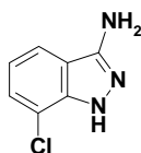
7-chloro-1H-indazol-3-amine
