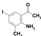
1-(2-amino-5-iodo-3-methylphenyl)-1-ethanone
